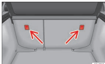
Fig. 25 Anilla de sujeción Top Tether*.
