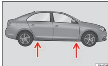
Fig. 63 Cambio de rueda: puntos de apoyo del gato.
