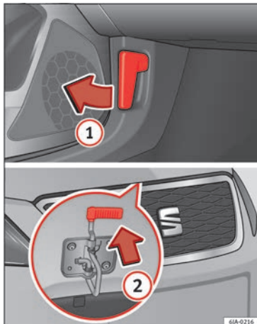
Fig. 7 Desbloqueo del capó del motor.
