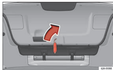
Fig. 6 Detalle del maletero: acceso al desbloqueo de emergencia.
