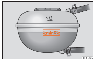
Fig. 226 En el vano delantero: marca en el depósito de expansión del líquido refrigerante.
