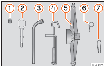
Fig. 209 En el maletero, bajo la cubierta de la superficie de carga: herramientas de a bordo.
