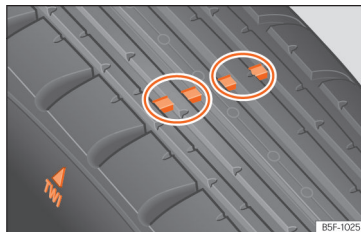
Fig. 239 Perfil del neumático: indicadores de desgaste.
