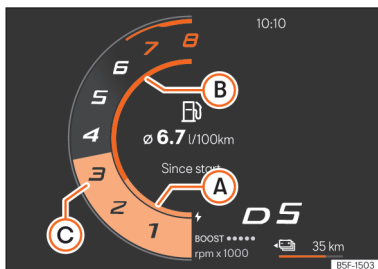
Fig. 5 Cuadro de instrumentos digital: Powermeter
