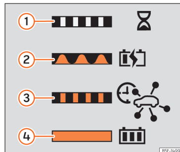
Fig. 62 En la cara interior de la tapa de la toma de carga de la batería: adhesivo con información sobre el indicador del proceso de carga.
