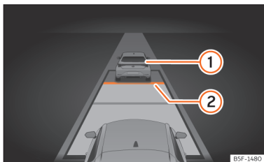
Fig. 136 En la pantalla del cuadro de instrumentos: ACC activo.
