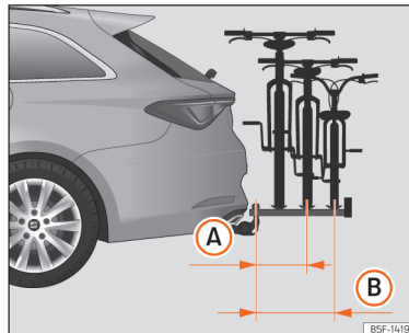
Fig. 203 Representación esquemática del voladizo máximo de la carga en un portabicicletas para dos o tres bicicletas.
