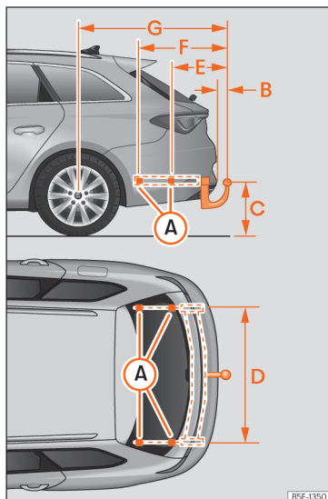
Fig. 204 Cotas y puntos de fijación para el montaje posterior de un dispositivo de remolque.
