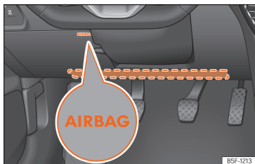
Fig. 35 En el lado del conductor: ubicación del airbag para las rodillas.
