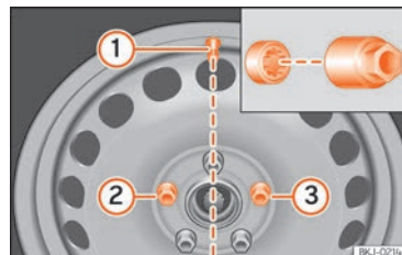
Fig. 227 Cambio de rueda: válvula del neumático ① y lugar de montaje del tornillo de rueda antirrobo ② o ③.
