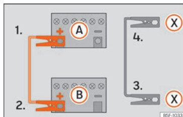
Fig. 194 Esquema de conexión para vehículos con sistema Start-Stop.
