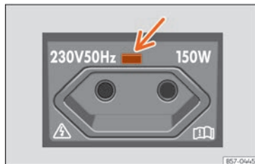
Fig. 157 En el lado izquierdo del maletero: toma de corriente de 230 voltios.
