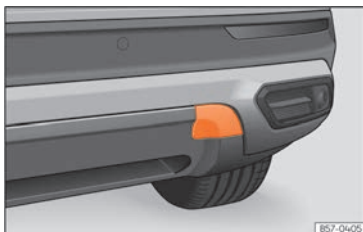
Fig. 199 En el lado derecho del paragolpes trasero: retirar la tapa.
