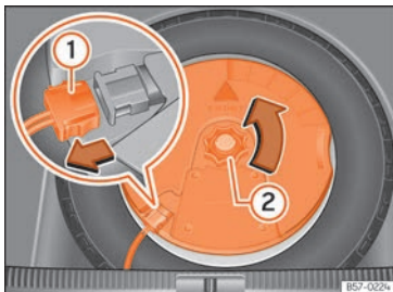
Fig. 222 En el maletero: desmontar el subwoofer.
