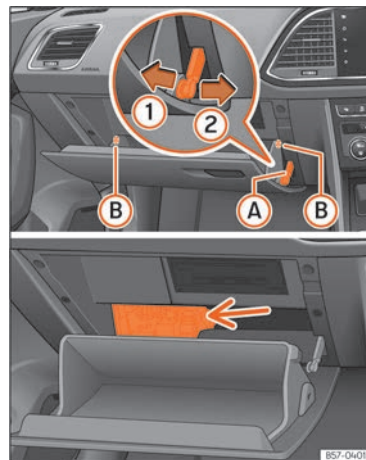
Fig. 202 Vehículos con el volante a la derecha: tapa de la caja de fusibles del tablero de instrumentos, en el lado del acompañante.
