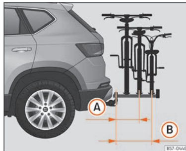
Fig. 184 Representación esquemática del voladizo máximo de la carga en un portabicicletas para dos o tres bicicletas.
