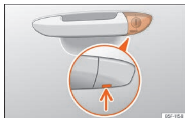
Fig. 52 Manecilla de la puerta del conductor: bombín de cierre oculto.
