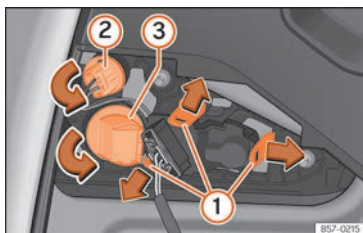
Fig. 206 Desmontar el portalámparas.
