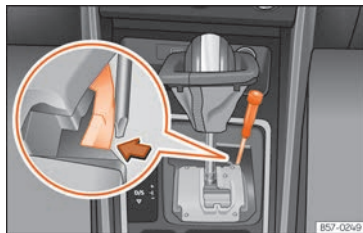
Fig. 101 Palanca selectora: desbloqueo de emergencia en la posición de aparcamiento.
