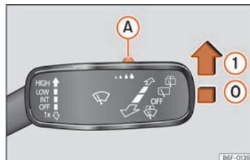
Fig. 84 Palanca del limpiaparabrisas: ajustar el sensor de lluvia A .
