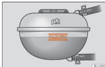
Fig. 180 En el vano delantero: marca en el depósito de expansión del líquido refrigerante.
