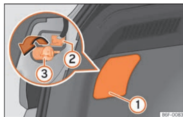
Fig. 171 Maletero: acceso al tornillo de fijación de la unidad de luz trasera.
