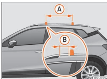
Fig. 148 Puntos de fijación de las barras transversales para el portaequipajes del techo
