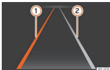
Fig. 111 En la pantalla del cuadro de instrumentos: indicaciones del sistema de aviso de salida del carril.
