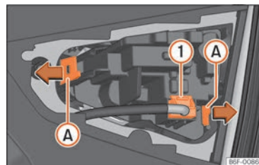
Fig. 174 Desmontar el portalámparas.
