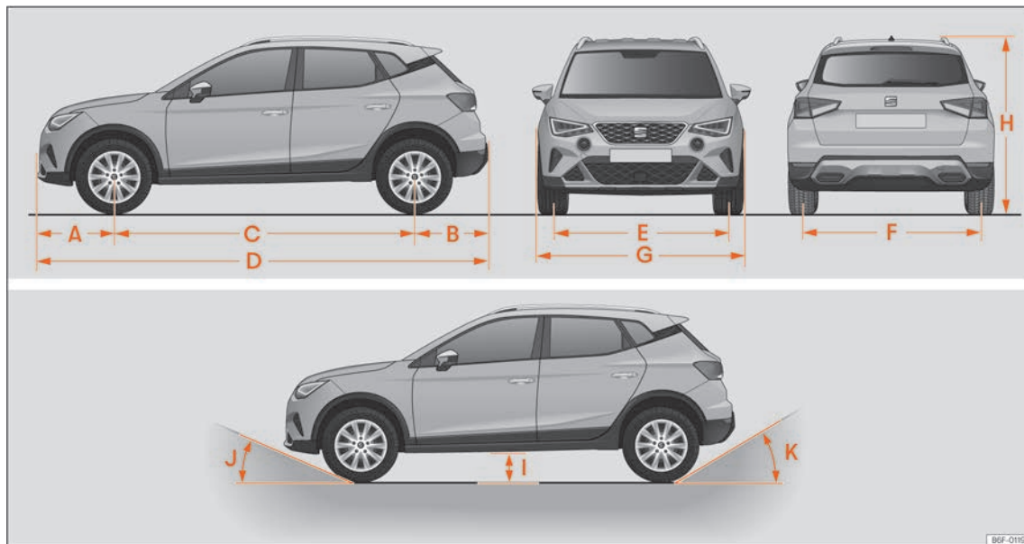
Fig. 206 Dimensiones y ángulos.
