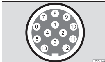
Fig. 149 Representación esquemática: asignación de los pines de la toma de corriente para remolque.
