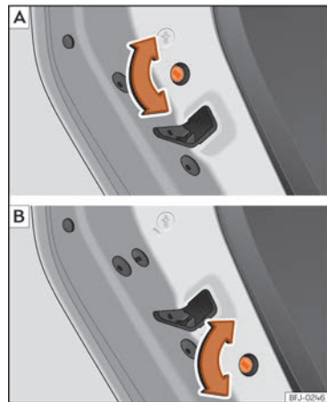
Fig. 54 Seguro para niños de la puerta izquierda (simétrico en la puerta derecha). En función de la versión o el país, el vehículo monta la variante A o bien la variante B .
