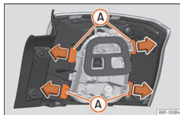
Fig. 172 Lengüetas de fijación en la parte posterior de la unidad de luz trasera.
