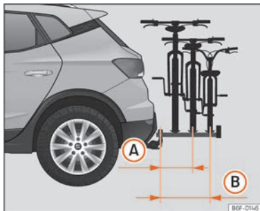
Fig. 151 Representación esquemática del voladizo máximo de la carga en un portabicicletas para dos o tres bicicletas.
