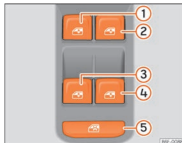
Fig. 57 Detalle de la puerta del conductor: mandos para las ventanillas.
