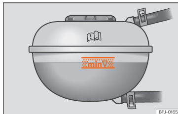
Fig. 221 A l'obertura davantera: marca al dipòsit d'expansió del líquid refrigerant.
