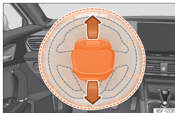
Fig. 30 Coixí de seguretat del conductor al volant.
