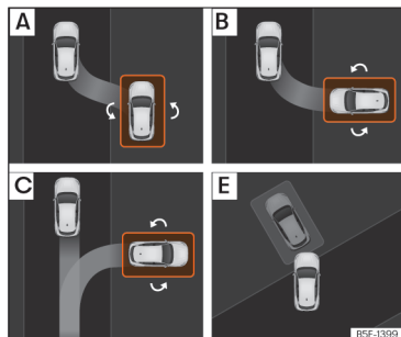
Fig. 152 A la pantalla del sistema d'Infotainment: indicació dels modes d'aparcament.
