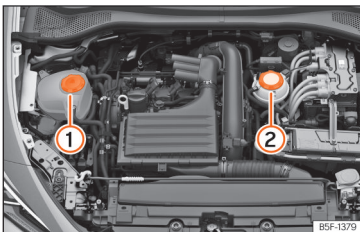
Fig. 220 Compartiment del motor: Dipòsit de líquid refrigerant
