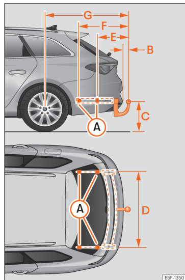
Fig. 201 Cotes i punts de fixació per al muntatge posterior d'un dispositiu de remolc.
