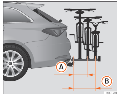
Fig. 200 Representació esquemàtica del voladís màxim de la càrrega en un portabicicletes per a dues o tres bicicletes.
