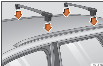
Fig. 195 Punts de fixació de les barres longitudinals per al portaequipatges del sostre (Leon Sportstourer).
