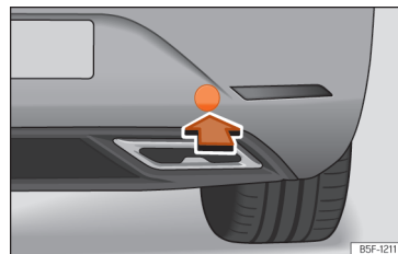
Fig. 213 A la part dreta del para-xocs del darrere: retirar la tapa.
