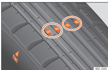
Fig. 233 Perfil del pneumàtic: indicadors de desgast.
