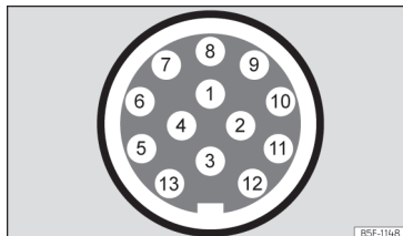
Fig. 197 Representació esquemàtica: assignació dels pins de l'endoll de corrent per a remolc.
