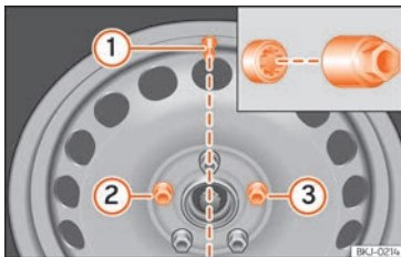
Fig. 44 Cambio de rueda: válvula del neumático ① y lugar de montaje del tornillo de rueda antirrobo ② o ③.
