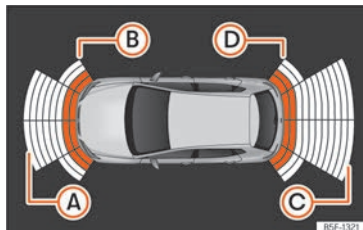
Fig. 203 Visualización de ayuda al aparcamiento en la pantalla del sistema de infotainment.
