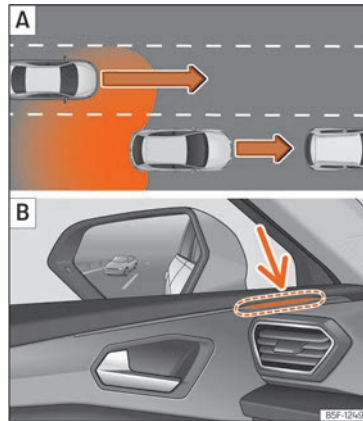
Fig. 191 Representación esquemática: A ) Situación en un adelantamiento con tráfico en la parte trasera. B ) Indicación del asistente de cambio de carril en el testigo de control del lado izquierdo.
