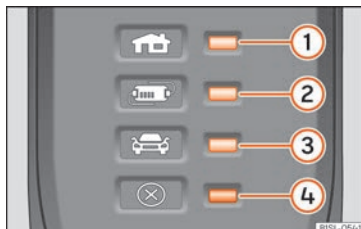
Fig. 219 En el cable de carga para tomas de corriente: Testigos de control en el dispositivo de protección.
