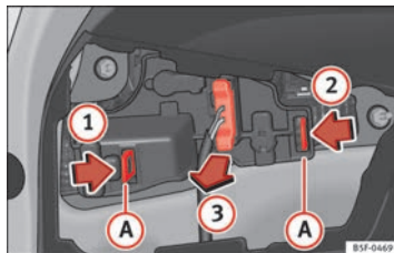
Fig. 200 Desmontar el portalámparas.
