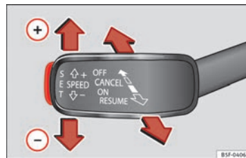
Fig. 131 A la izquierda de la columna de la dirección: tercera palanca de 6 posiciones para el mando del GRA.
