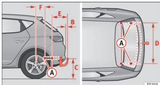
Fig. 157 Puntos de fijación del dispositivo de remolque.
