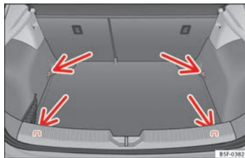
Fig. 106 En el maletero: argollas de amarre (modelo LEON/LEON SC excepto versiones con rueda de recambio de dotación y GNC).
