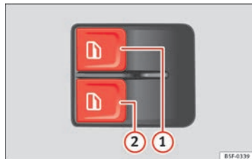
Fig. 61 Detalle de la puerta del conductor: mandos para las ventanillas (vehículo con elevallunas eléctricos anteriores).
