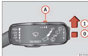
Fig. 75 Palanca del limpiaparabrisas: ajustar el sensor de lluvia A.
