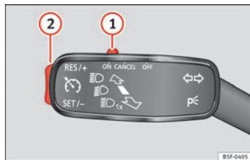
Fig. 130 A la izquierda de la columna de la dirección: conmutador y mandos de manejo del GRA.
