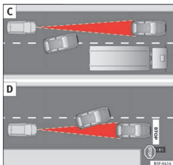
Fig. 140 (C) Cambio de carril de un vehículo. (D) Vehículo girando y otro detenido.
