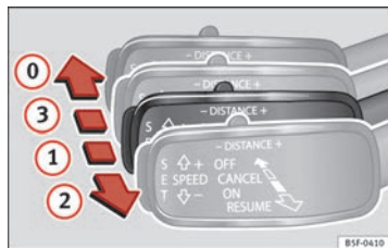
Fig. 137 A la izquierda de la columna de la dirección: tercera palanca para manejar el control adaptativo de velocidad.
