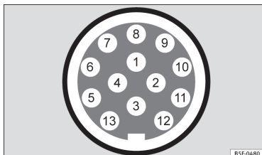
Fig. 156 Representación esquemática: asignación de los pines de la toma de corriente del remolque.
