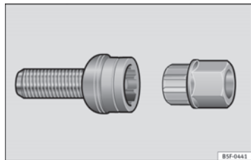
Fig. 171 Tornillo antirrobo de la rueda con capuchón y adaptador.
