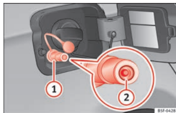
Fig. 159 Tapa del depósito abierta: boca de carga de gas ①, retén de la boca de carga ②.
