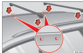
Fig. 115 Leon ST: puntos de fijación de las barras longitudinales para el portaequipajes del techo. ►
