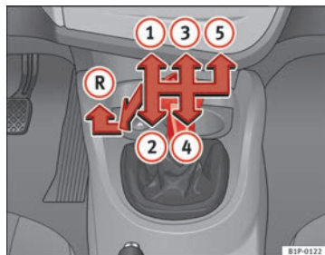
Fig. 121 Detalle de la consola central: esquema de un cambio manual de 5 marchas
