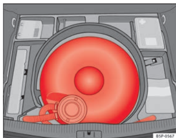
Fig. 140 Depósito de GLP en la cavidad de la rueda de repuesto.
