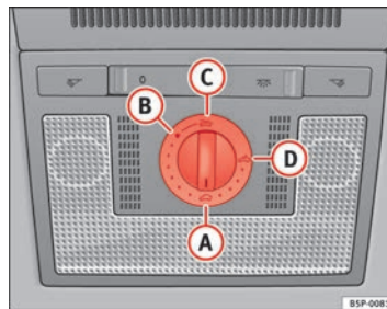
Fig. 69 Detalle del revestimiento interior del techo: mando giratorio del techo corredizo/ deflector
