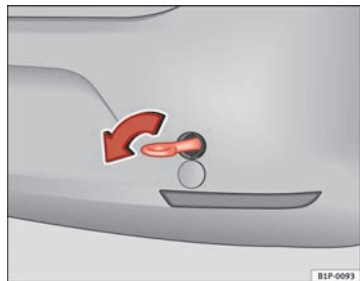
Fig. 183 Atornillado de la argolla de remolque en la parte trasera del vehículo
