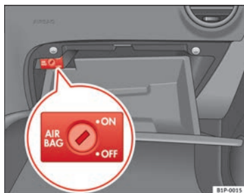
Fig. 25 En la guantera: conmutador con llave para activar y desactivar el airbag del acompañante
