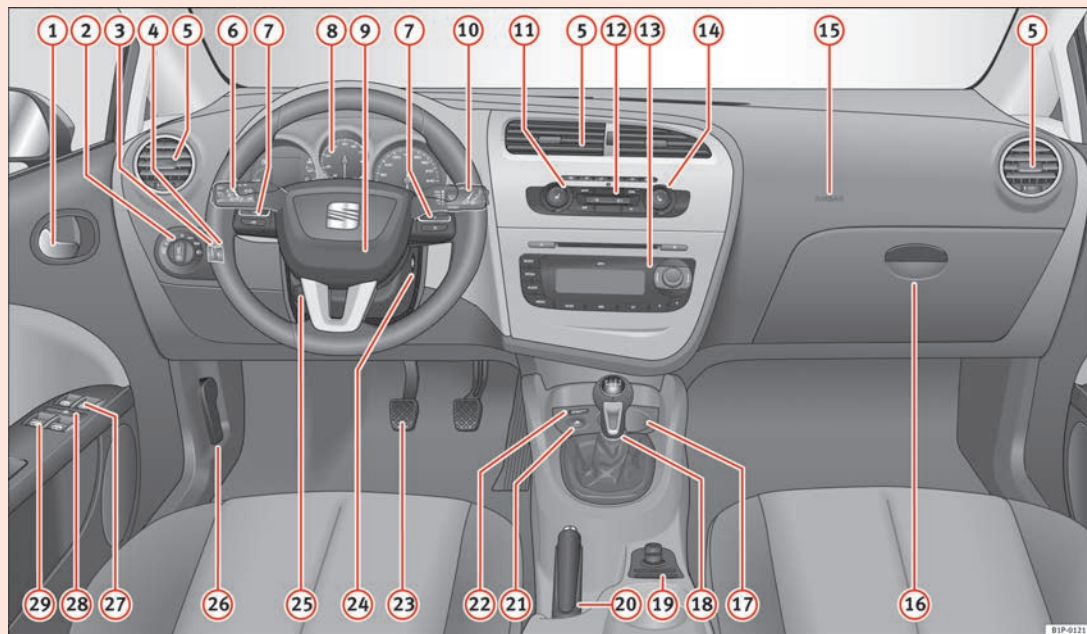
Fig. 31 Tablero de instrumentos
