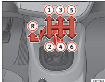
Fig. 122 Detalle de la consola central: esquema de un cambio manual de 6 marchas
