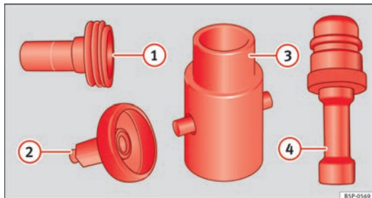
Fig. 141 Cuadro general de los adaptadores para la boca de carga de GLP.
