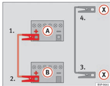
Fig. 181 Esquema para conectar los cables de emergencia en el caso de que el vehículo que suministra la corriente disponga del sistema Start-Stop: batería descargada (A) y batería que suministra la corriente (B).
