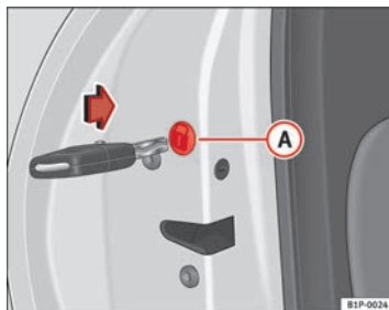
Fig. 58 Cierre de emergencia de las puertas
