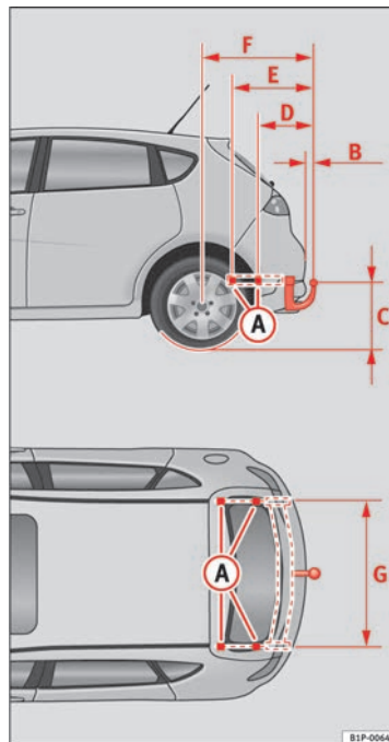
Fig. 137 Puntos de fijación del dispositivo de remolque
