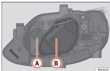
Fig. 99 Lámparas del faro AFS.
