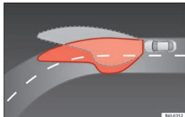
Fig. 126 Iluminación de la curva con faros autodireccionables.
