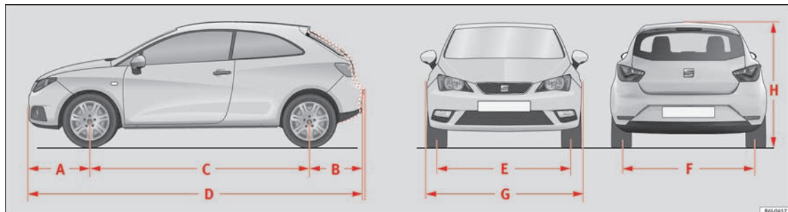
Fig. 182 Dimensiones
