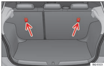
Fig. 26 Posición de las anillas Top Tether en la parte posterior del asiento trasero.
