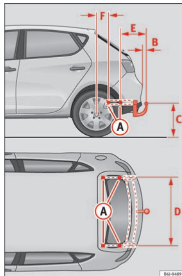
Fig. 172 IBIZA/IBIZA SC: puntos de fijación del dispositivo de remolque.
