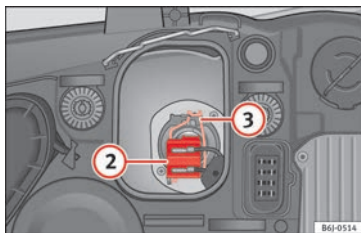
Fig. 97 Luz de cruce.
