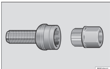
Fig. 63 Tornillo antirrobo de la rueda con capuchón y adaptador.
