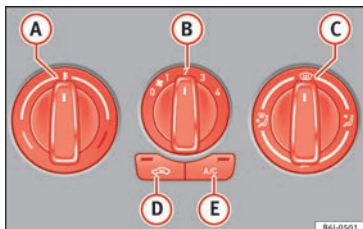
Fig. 48 En la consola central: mandos del aire acondicionado manual.
