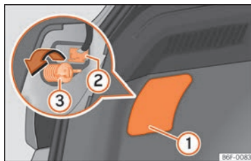
Fig. 170 Maletero: acceso al tornillo de fijación de la unidad de luz trasera.
