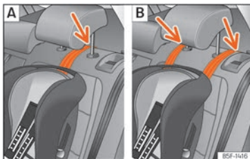
Fig. 40 Asientos traseros: ajuste y montaje en función del cinturón Top Tether.
