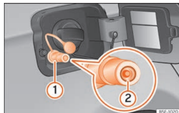
Fig. 155 Tapa del depósito abierta: boca de carga de gas (1), retén de la boca de carga (2).
