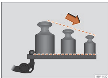
Fig. 149 Reparto recomendado del peso en el sistema portante trasero.
