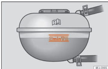
Fig. 179 En el vano delantero: marca en el depósito de expansión del líquido refrigerante.
