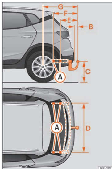
Fig. 151 Cotas y puntos de fijación para el montaje posterior de un dispositivo de remolque.
