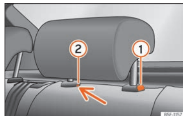
Fig. 69 Apoyacabezas trasero: desmontaje.
