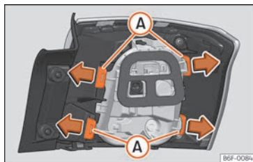
Fig. 171 Lengüetas de fijación en la parte posterior de la unidad de luz trasera.
