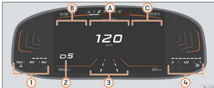
Fig. 3 Cuadro de instrumentos digital versión Basic: Vista principal.
